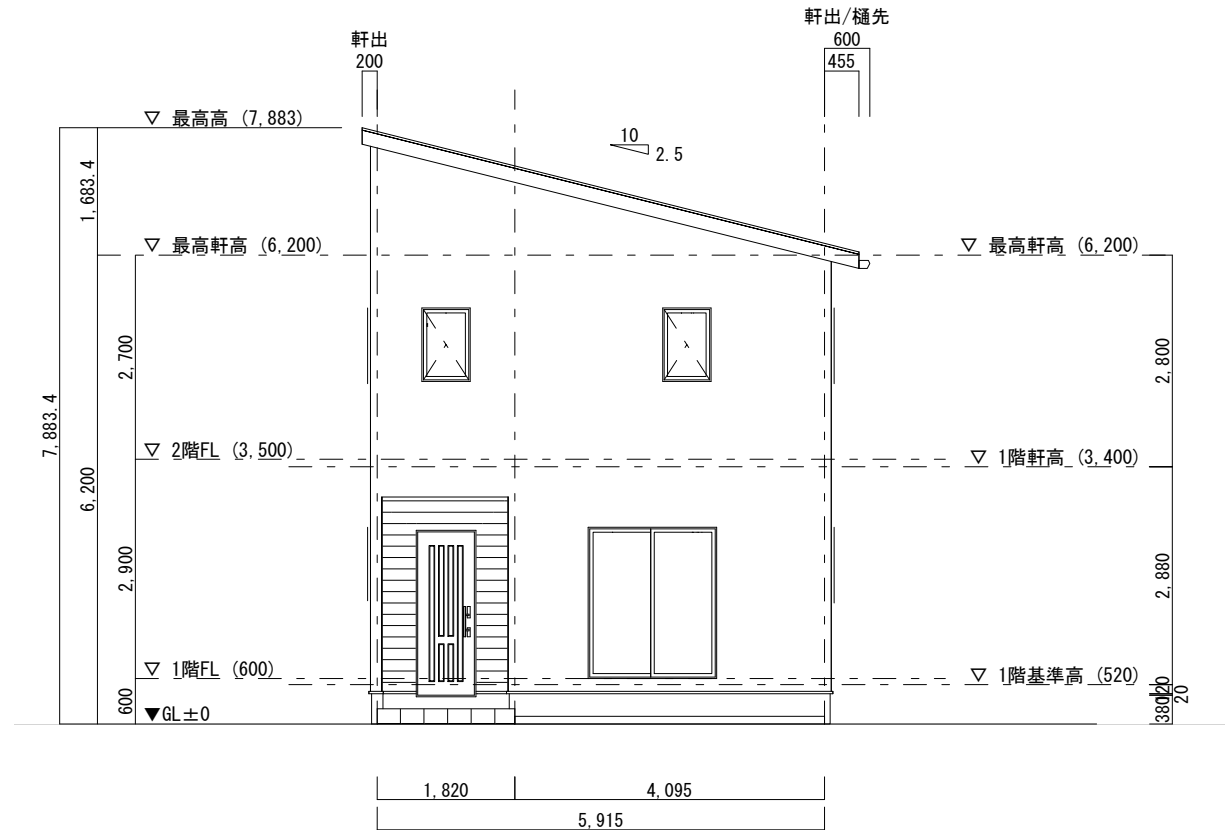
立面図-西側(図面)
